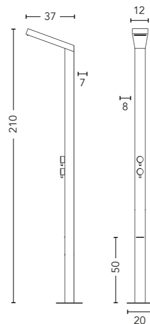
DIMENSÕES 12cm x 37cm x 210cm (larg./prof./alt.)
