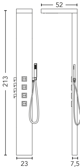
DIMENSÕES COLUMNA 23cm x 52cm x 213cm (larg./prof./alt.)
